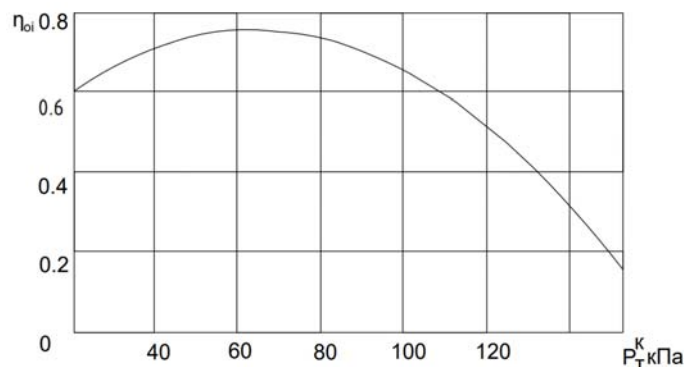
Рисунок 1 – Зависимость относительного внутреннего КПД \eta_{0i} турбины Т-110-120-130 ЛМЗ, от давления p_T^H в нижнем отопительном отборе (ст. № 23 (ЦСД))
