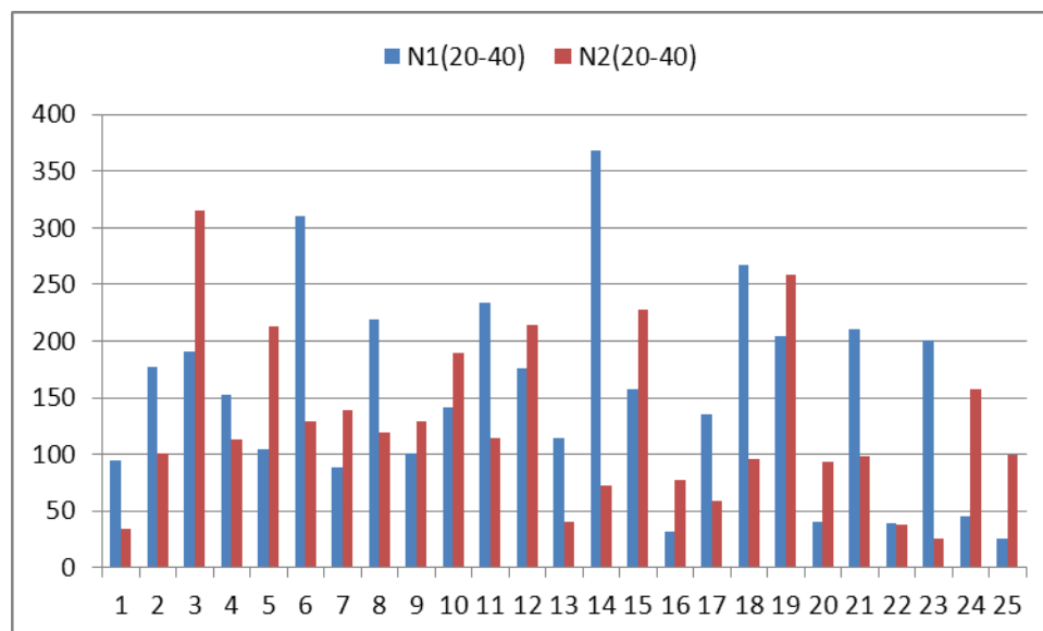
Рисунок 5. Результативность движения робота в диапазоне Range((20,20):( 40,40))
