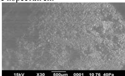
1 - Сурет. Сібір самырсын жаңғағы қабығының ұнтағының микроқұрылымды талдауы
