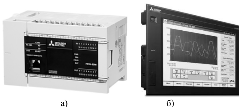
Сурет 3. Mitsubishi MELSEC iQ-F сериясының а - FX5U-32M өнеркәсіптік контроллері және Mitsubishi GOT 2000 сериялы б - GT 27 HMI панелі
