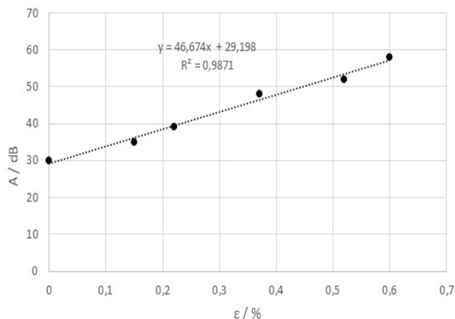
Рисунок 4. График роста дополнительных потерь световой волны при росте относительной деформации балки
