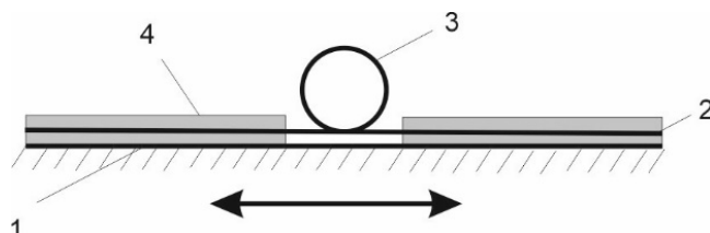
Рисунок 3. Конструкция петли из оптического волокна (сенсор): 1- боковая грань балки, 2 – оптическое волокно, 3 – петля из оптического волокна (сенсор), 4 – слой эпоксидного клея
