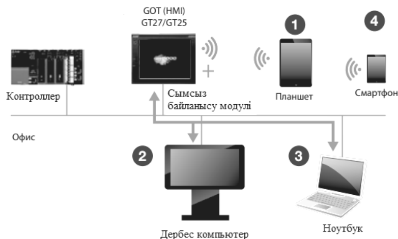
Сурет 7. GOT mobile функциясына қосылу сұлбасы
