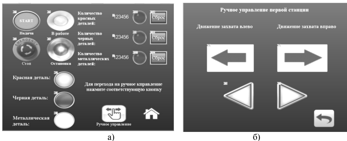
Сурет 4. HMI GOT 2000 оператор панелінің басты басқару терезелері: а – автоматты басқару; б – қолмен басқару.
