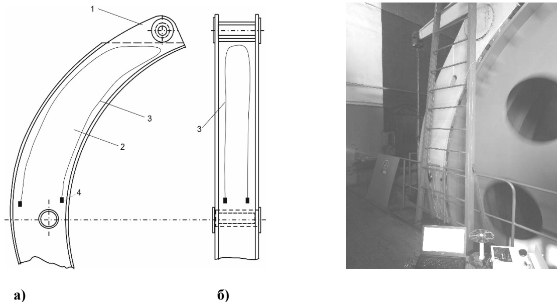
Рисунок 1. Варианты размещения оптического волокна на боковых гранях металлической конструкции балки тормозного устройства: 1- проушина для крепления втулки, 2 – балка тормозного устройства, 3 – оптическое волокно (сенсор). а – схема размещения, б – фото проведения эксперимента и установка измерительных приборов.
