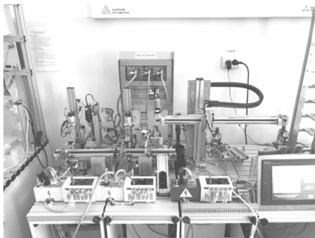
Сурет 1. «FESTO мехатрондық желісі» стендінің жалпы көрінісі
