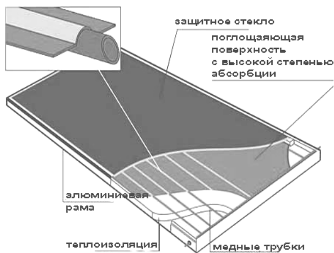
Рисунок 2 - Структура PV-T коллектора
