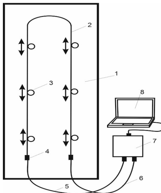
Рисунок 2. Схема проведения измерений: 1- боковая грань балки, 2 – оптическое волокно, 3 – петли из оптического волокна (сенсор), 4 – коннектор, 5, 6 - оптические патч-корд 7 - блоком обработки данных, 8 - ноутбуке.
