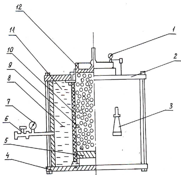
6 – сурет. Эксперименттік стабилометрдің схемасы.
