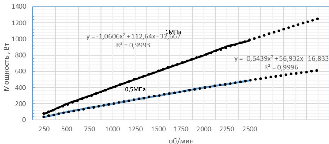
Рисунок 2 – Зависимость развиваемой механической мощности от числа оборотов коленчатого вала при различных значениях давления 1 МПа и 0,5 МПа
