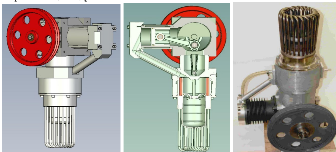
Рисунок 1 –Лабораторный образец ДС и 3 D модель.
