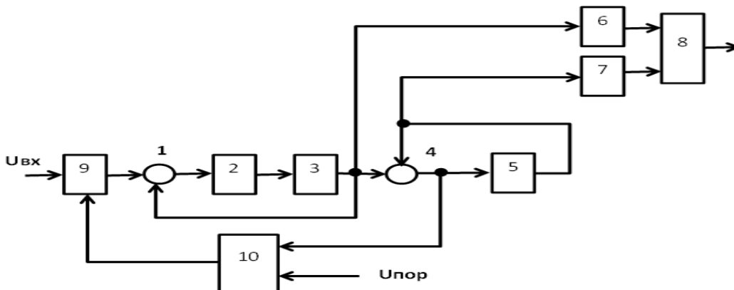
Рисунок 3 – Электрическая схема сглаживающего устройства
