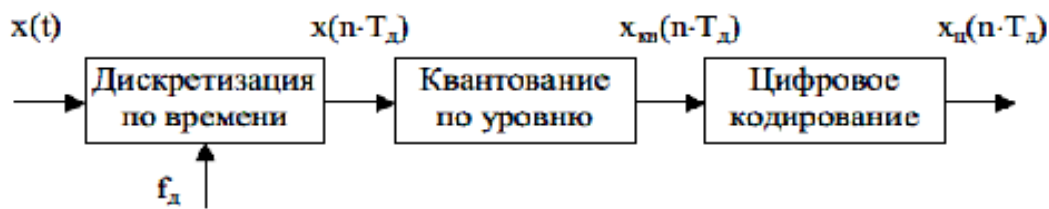
Рисунок 1 – Аналого-цифровое преобразование сигнала
