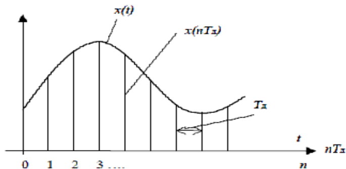
Рисунок 2 - График непрерывного x(t) и дискретного x(nT_D) сигнала
