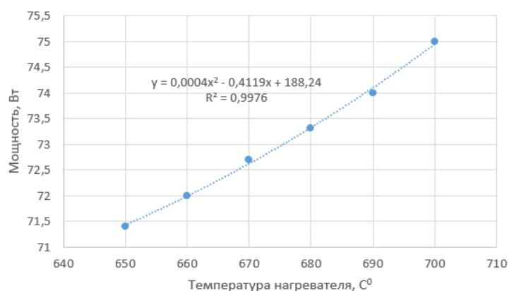
Рисунок 4 - Зависимости полученной механической мощности на валу в зависимости от изменения температуры нагревателя
