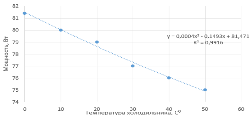
Рисунок 2 - Зависимости полученной механической мощности на валу в зависимости от изменения температуры холодильника
