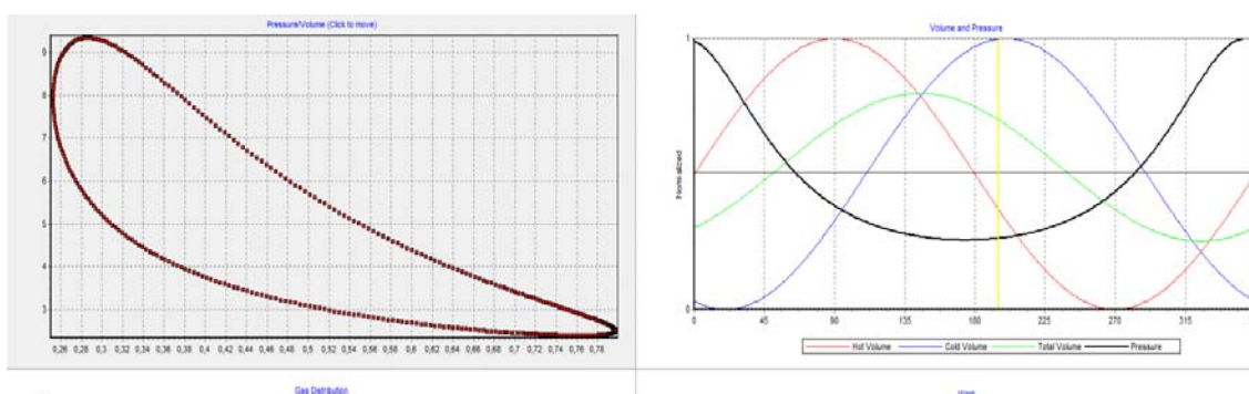
Рисунок 3 - Результат моделирования при изменении температуры холодильника от 0 до 60 С 0
