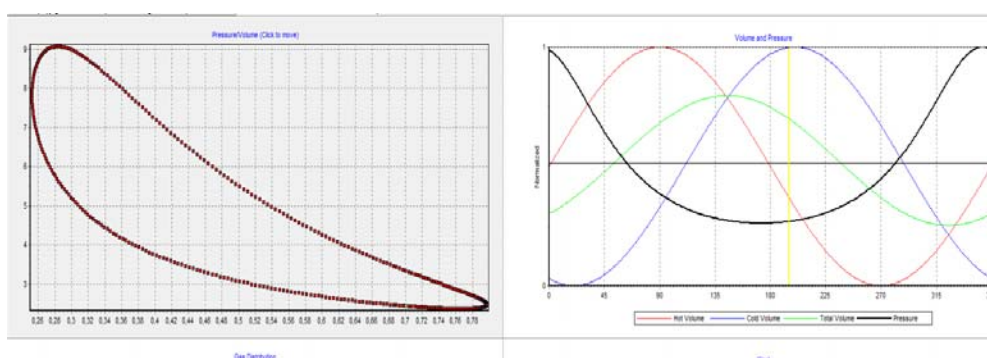
Рисунок 5 - Результат моделирования при изменении температуры нагревателя от 650 до 700 С 0
