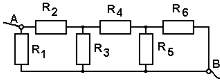
3 сурет – Электрлік тізбек
