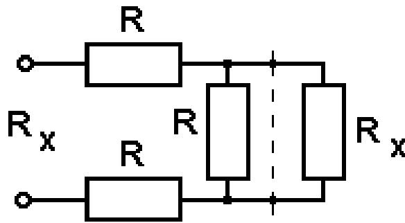
2 сурет – Шексіз тізбек кедергілері
