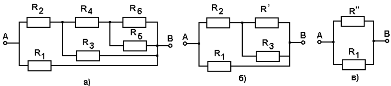
4 сурет – Эквивалентті тізбек құрастыру
