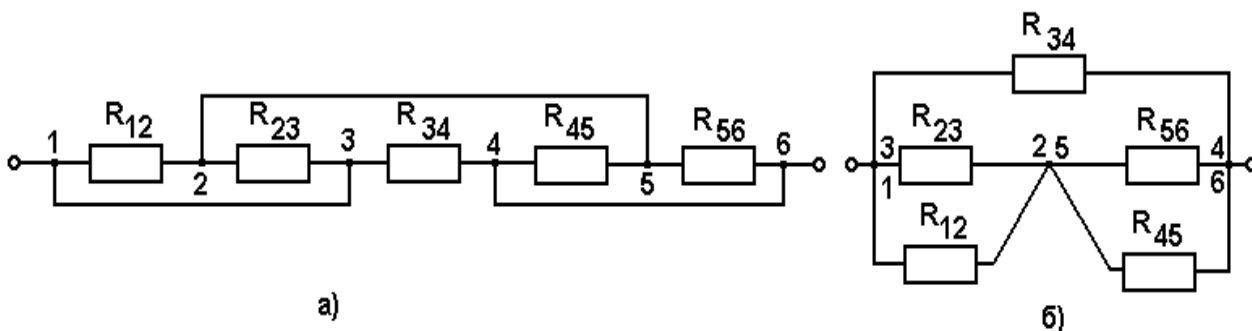
5 сурет – Тізбектің эквивалентті нұсқасын алу.
