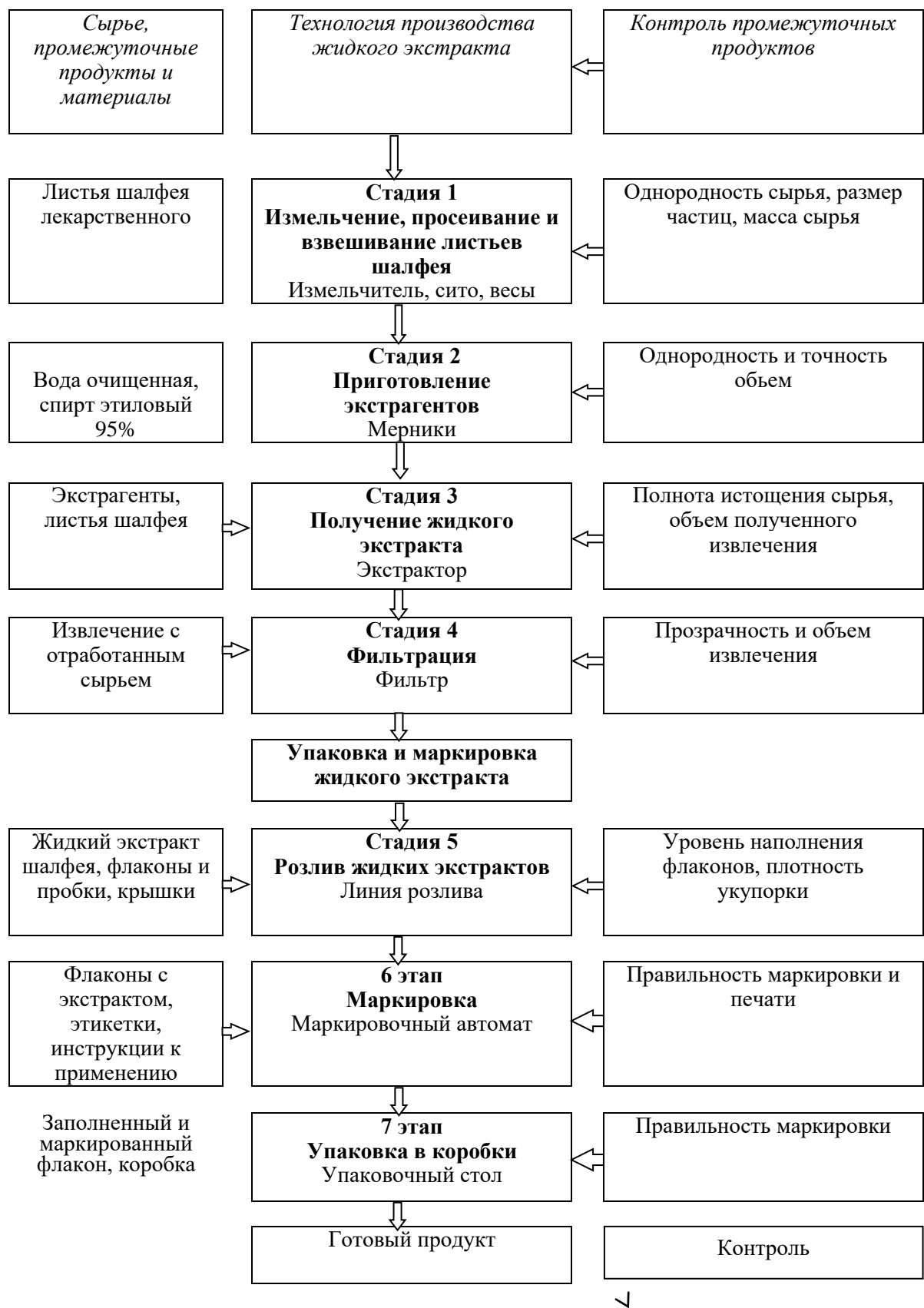
Технологическая схема производства ультразвукового экстракта Salvia officinalis
