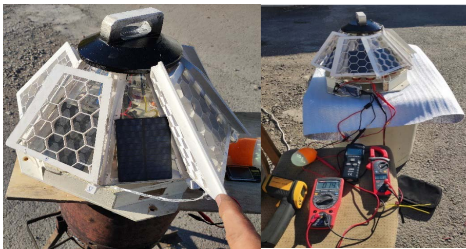
Рисунок 2 - Внешний вид модели ГВСЭ
