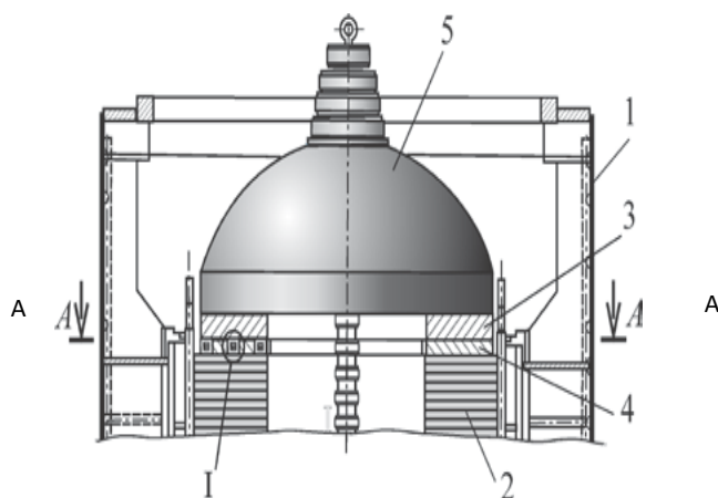
Сурет 1. Престегі қосымша қысым сақинасын орнату схемасы: 1-статор корпусы; 2-статор өзегі; 3 - жоғарғы қысым сақинасы; 4 - төменгі қысым сақинасы; 5 – пресс
