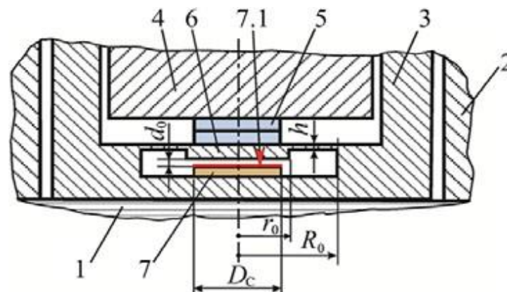
Сурет 4. Сыйымдылық датчигының мембранасы мен электродтарының күйі: 1-статор өзегі; 2-төменгі қысым сақинасы; 3-клип; 4-втулка; 5-сынама; 6-мембрананың қатты орталығы; 7-диэлектрлік пластина; 7-сыйымдылық датчигының электроды; R_0 -мембрананың сыртқы радиусы; r_0 -мембрананың қатты центрінің радиусы; h -мембрананың қалыңдығы; D_c -электродтың диаметрі; d_0 -сыйымдылық датчигының диаметрі
