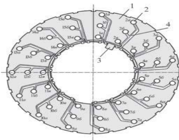
Сурет 2. Қосымша сақинаның жалпы көрінісі: 1 - металл диск; 2-бақылау ұяшығы; 3-кабельдер; 4-электрондық тіркеу блогы және өлшеу апаратын өңдеу
