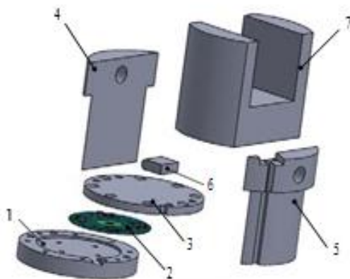
Сурет 6. CAD-бақылау ұяшығының моделi: 1-түбi; 2-сыйымдылықты түрлендiргiш; 3-мембрана;4-сол жақ тiрек; 5-оң жақ тiрек; 6-үлгi; 7-втулка
