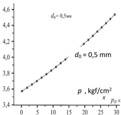
Сурет 7. Түрлендiргiштiң есептiк сипаттамасы
