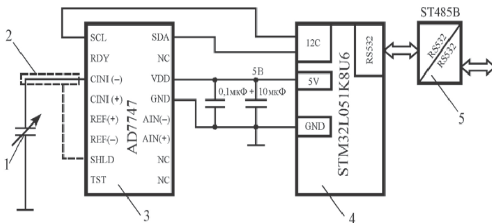
Сурет 5. Екiншi реттiк өлшеу түрлендiргiшiнiң схемалық электр схемасы: 1-ауыспалы жазықтық параллельдi жұмыс конденсаторы; 2-жұмыс конденсаторын паразиттiк ұштардан қорғауға арналған экран; 3-24 биттiк түрлендiргiш;4-микроконтроллер; 5-интерфейс түрлендiргiшi
