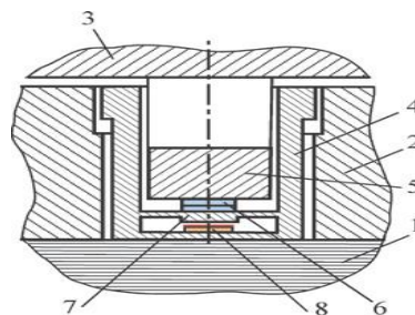
Сурет 3. Бақылау ұяшығының схемасы және оны орнату әдісі: 1-статор өзегі; 2-төменгі қысым сақинасы; 3-жоғарғы қысым сақинасы; 4-клип; 5-втулка; 6-бақылау қорғасын сынағы; 7-жалпақ мембрана ортасы; 8-жұқа пленкалы диэлектрлік пластинасы
