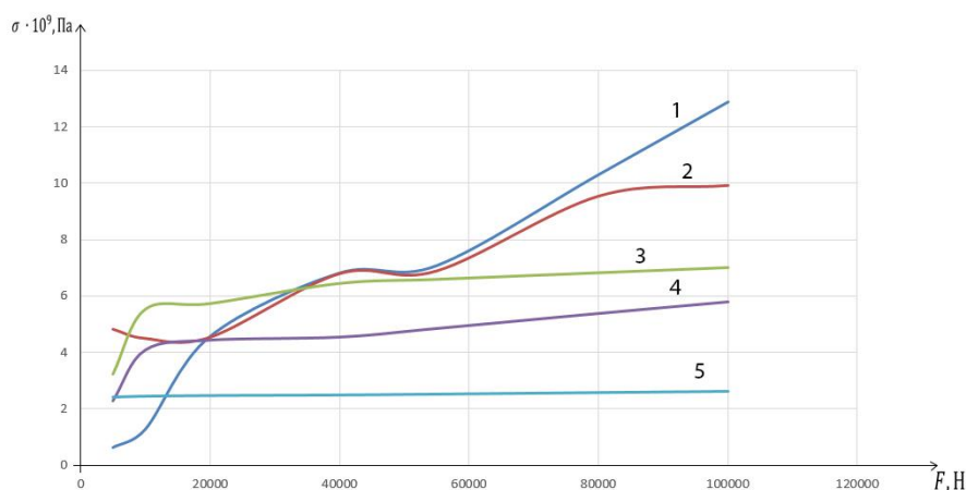
Рисунок 2 – Графики зависимости механического напряжения от нагрузки для направляющих устройств различных диаметров: 1 – d = 40 мм; 2 – d = 50 мм; 3 – d = 60 мм; 4 – d = 70 мм; 5 – d = 80 мм
